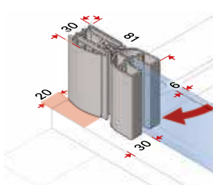
Hinge door part
