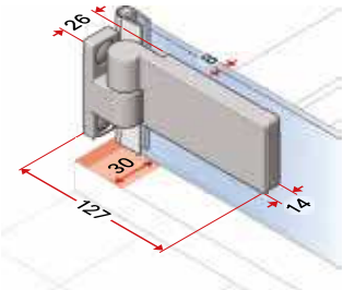
Hinge door part
