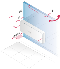
Door panel fixation side
