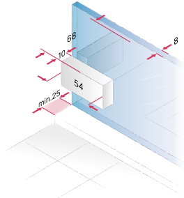
Pannello fisso e pannello laterale
