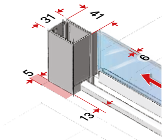
Serratura parte porta
