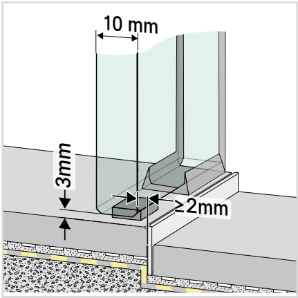
Sezione trasversale situazione di installazione terreno, battuta a sinistra
