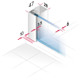
Parte fissa e parte laterale
