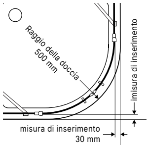
Dimensioni di montaggio
