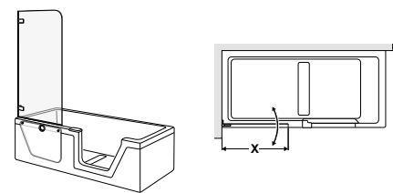
Panoramica, battuta a sinistra Vista dall'alto, battuta a sinistra
