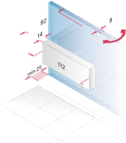
Battuta della porta
