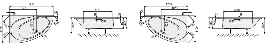
Vista dall'alto 600.470000 Panoramica 600.470000 Vista dall'alto 600.471000 Panoramica 600.471000
