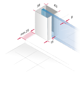
Pannello fisso e pannello laterale, profilo a parete
