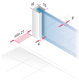
Pannello fisso e pannello laterale, profilo a parete
