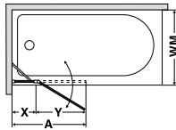
Vista dall'alto, battuta a sinistra
