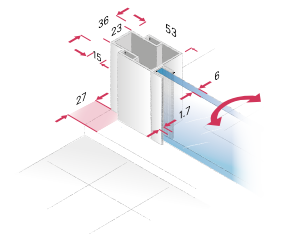
Serratura Parte porta
