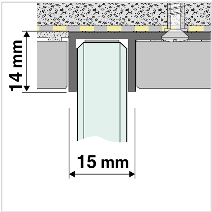
Dimensioni profilo a parete da incasso 520367
