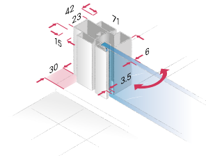
Fermo porta
