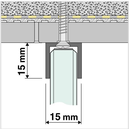
Dimensioni profilo per montaggio a parete 520369
