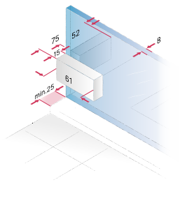
Pannello fisso e pannello laterale
