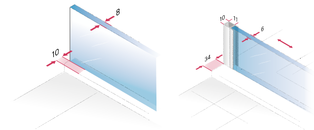
Porte fissa e parte laterale
