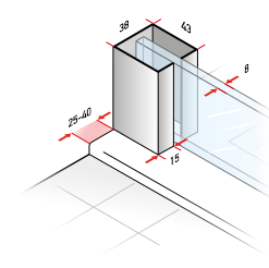
Parte fissa e parte laterale con profilo a parete
