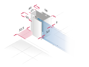
Parte fissa e parte laterale
