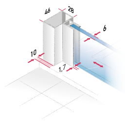
Serratura parte porta
