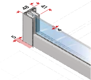
Pannello fisso, pannello laterale
