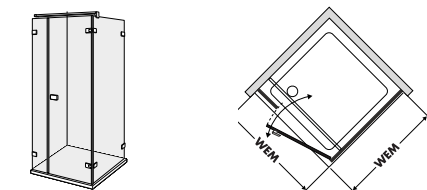
Panoramica, battuta a destra
