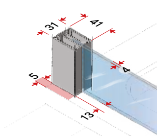
Pannello fisso e pannello laterale
