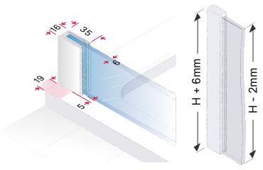
Pannello fisso e pannello laterale
