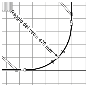
Dimensioni di montaggio
