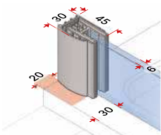
Pannello fisso/pannello laterale
