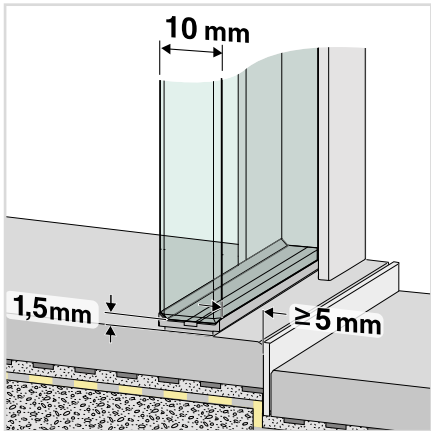
Montaggio trasversale profilo del pavimento, battuta a sinistra
