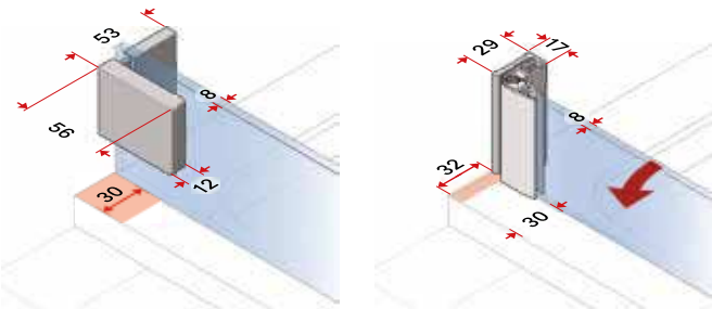
Pannello fisso/pannello laterale
