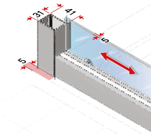
Chiusura della porta
